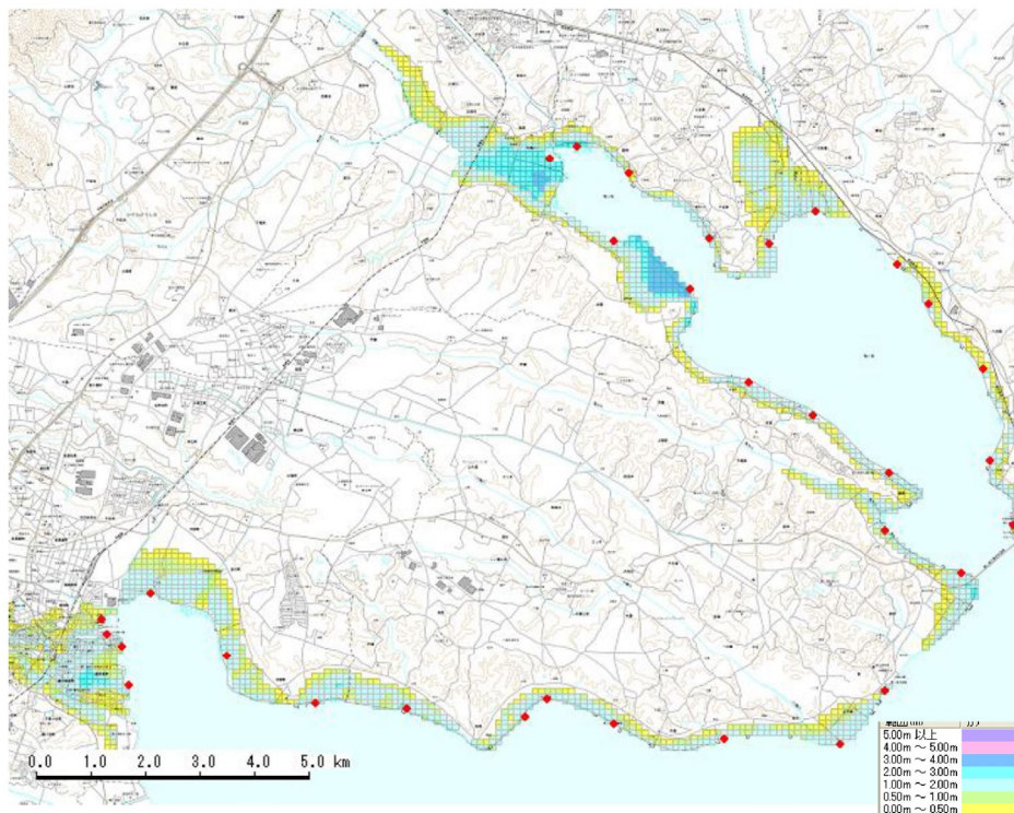
図 霞ヶ浦湖岸破堤想定による最大浸水の状況
