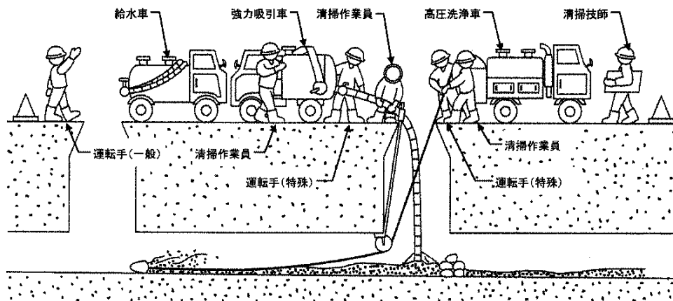
高圧洗浄車清掃工の作業模式図
