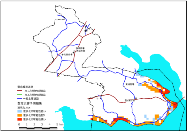
【かすみがうら市内の液状化危険度分布】
