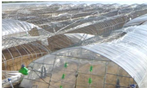
台風第15号で被災したパイプハウス
