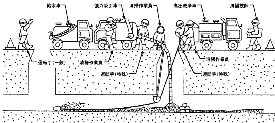
高压洗浄車清掃工の作業模式図
