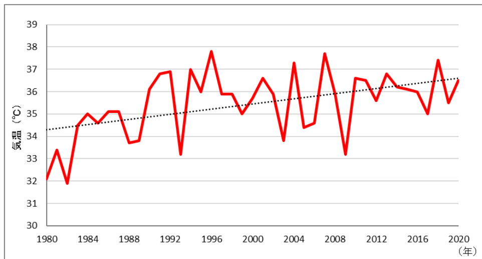
日最高気温の年間最高値経年変化（昭和55（1980）年～令和2（2020）年）
