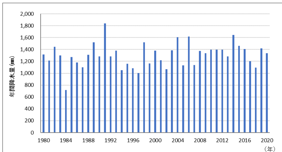
年降水量の経年変化（昭和55（1980）年～令和2（2020）年）
