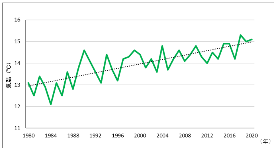
年平均の経年変化（昭和55（1980）年～令和2（2020）年）
