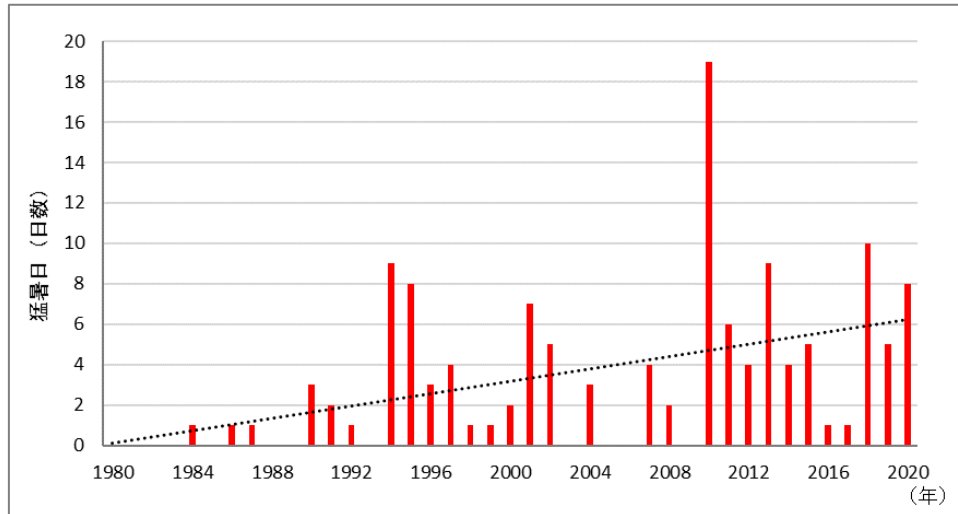
猛暑日数日の経年変化（昭和55（1980）年～令和2（2020）年）
