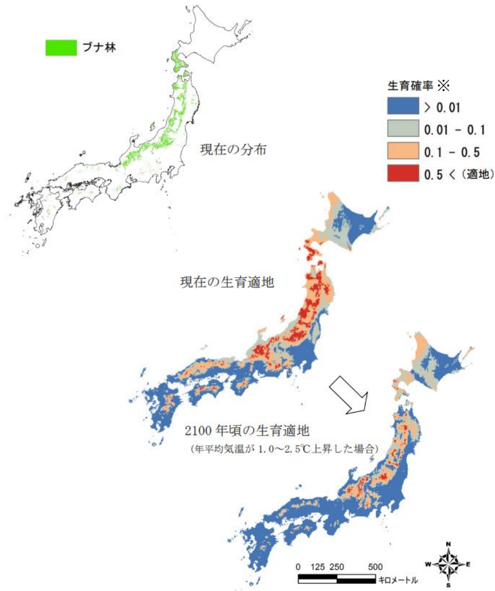
ブナ林の将来生育地予測
