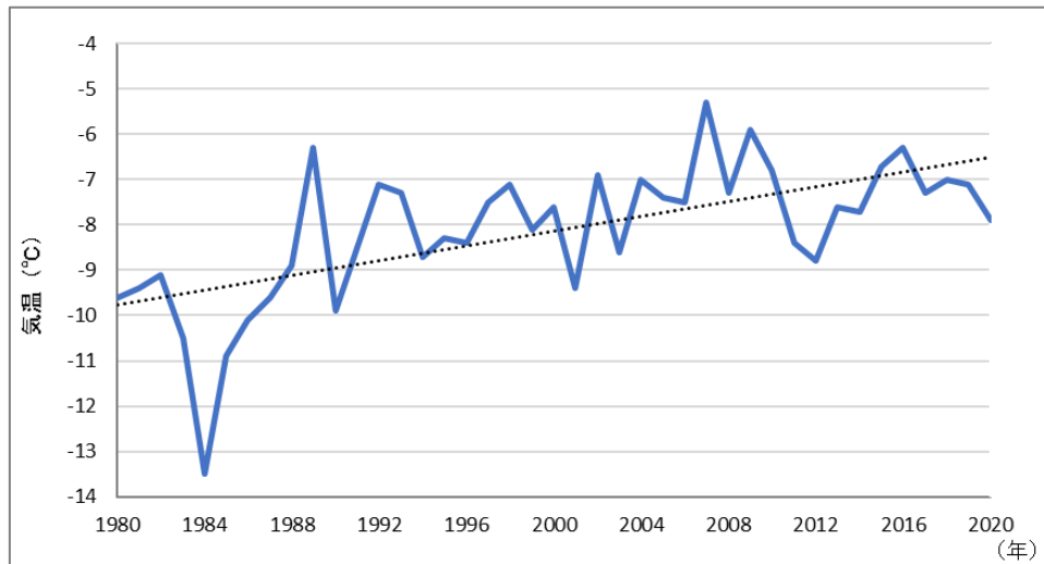
日最低気温の年間最低値経年変化（昭和55（1980）年～令和2（2020）年）
