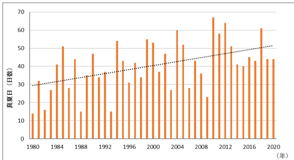
真夏日日数の経年変化（昭和55（1980）年～令和2（2020）年）
