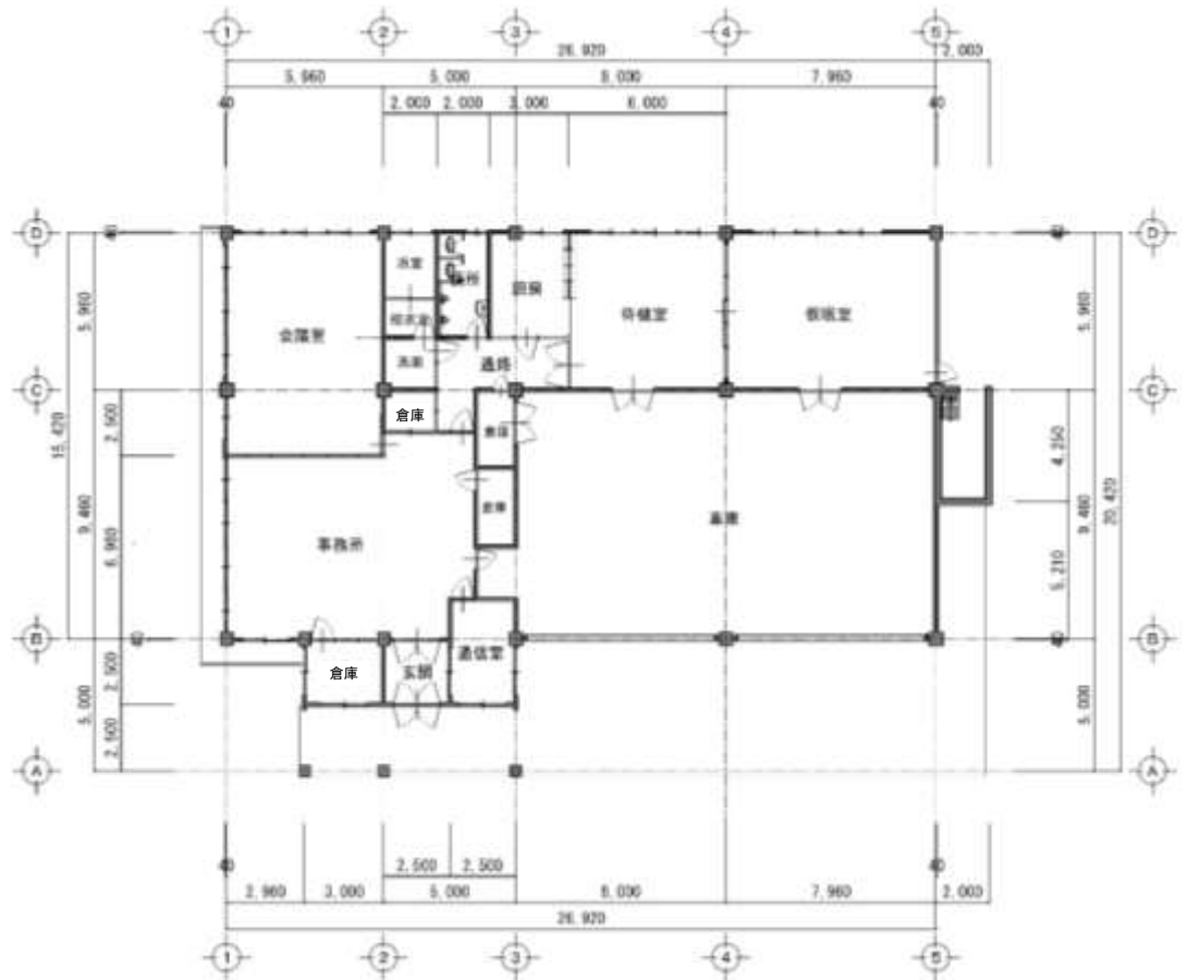
1階平面図
