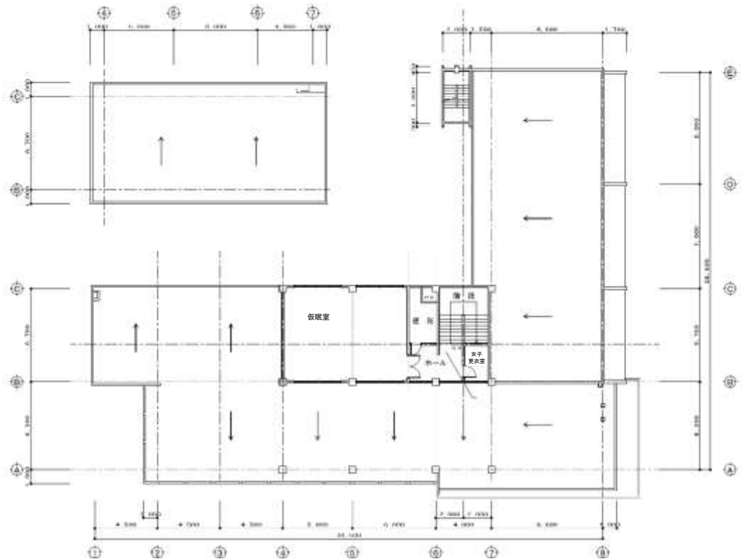
2階平面図
