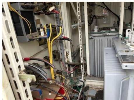
高圧受変電設備内部の損壊
