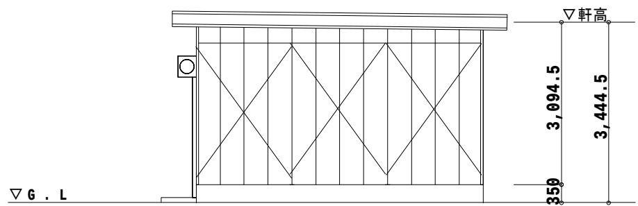
立 面 図
