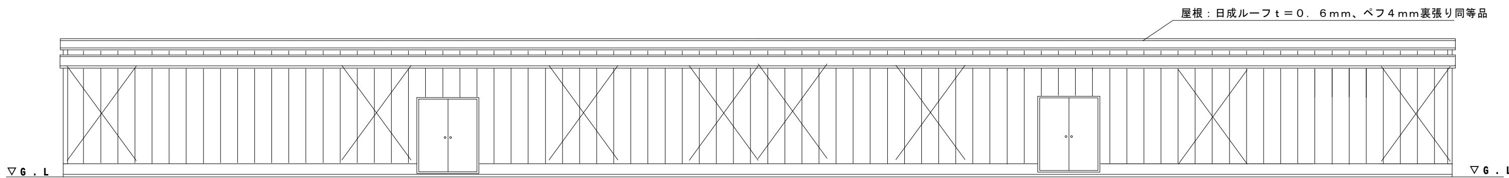
立 面 図
