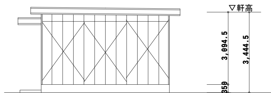
立 面 図
