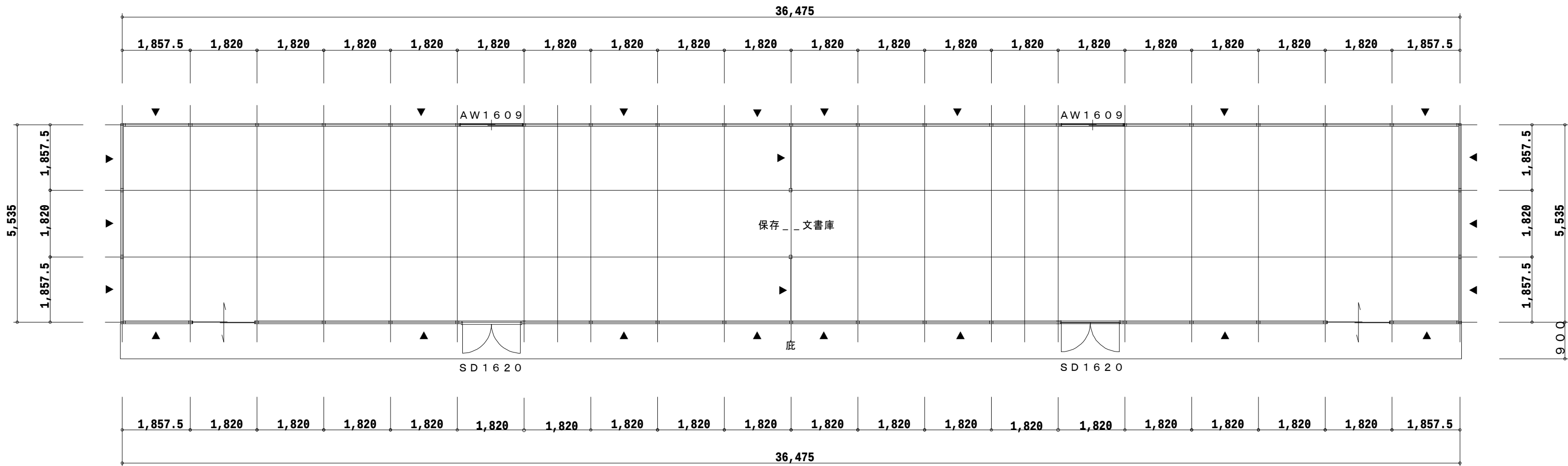
1 階平面図 各室面積 2 0 1 . 8 9 m 2
