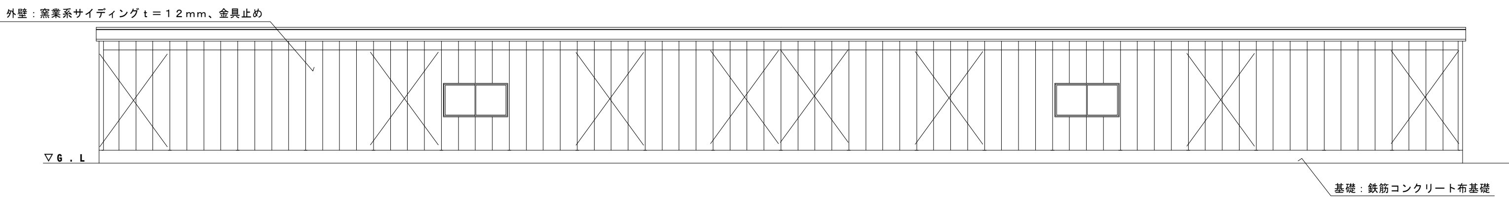
立 面 図
