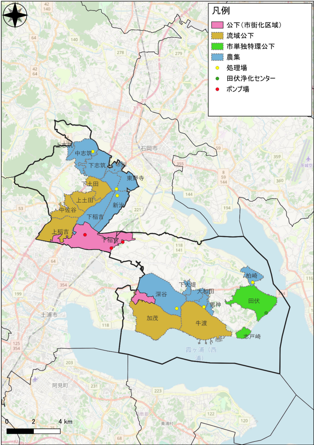
図 4.7.1 下水道処理区分概要図
