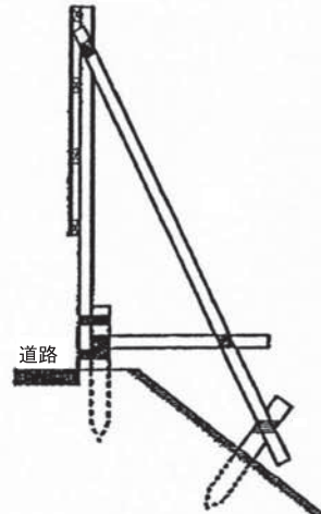
擁壁方式
